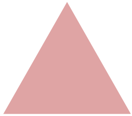
TRIÁNGULO
