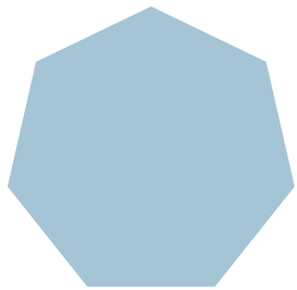
HEPTÁGONO
