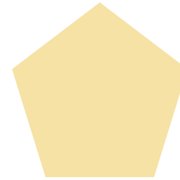
PENTÁGONO
