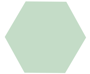
HEXÁGONO
